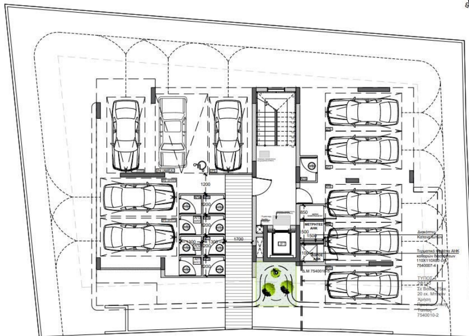
ΚΑΤΟΨΗ ΙΣΟΓΕΙΟΥ
