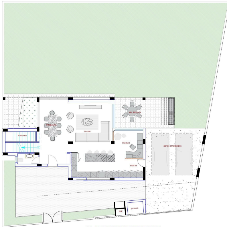
ΚΑΤΟΨΗ ΙΣΟΓΕΙΟΥ Κ.Α. 1:100
